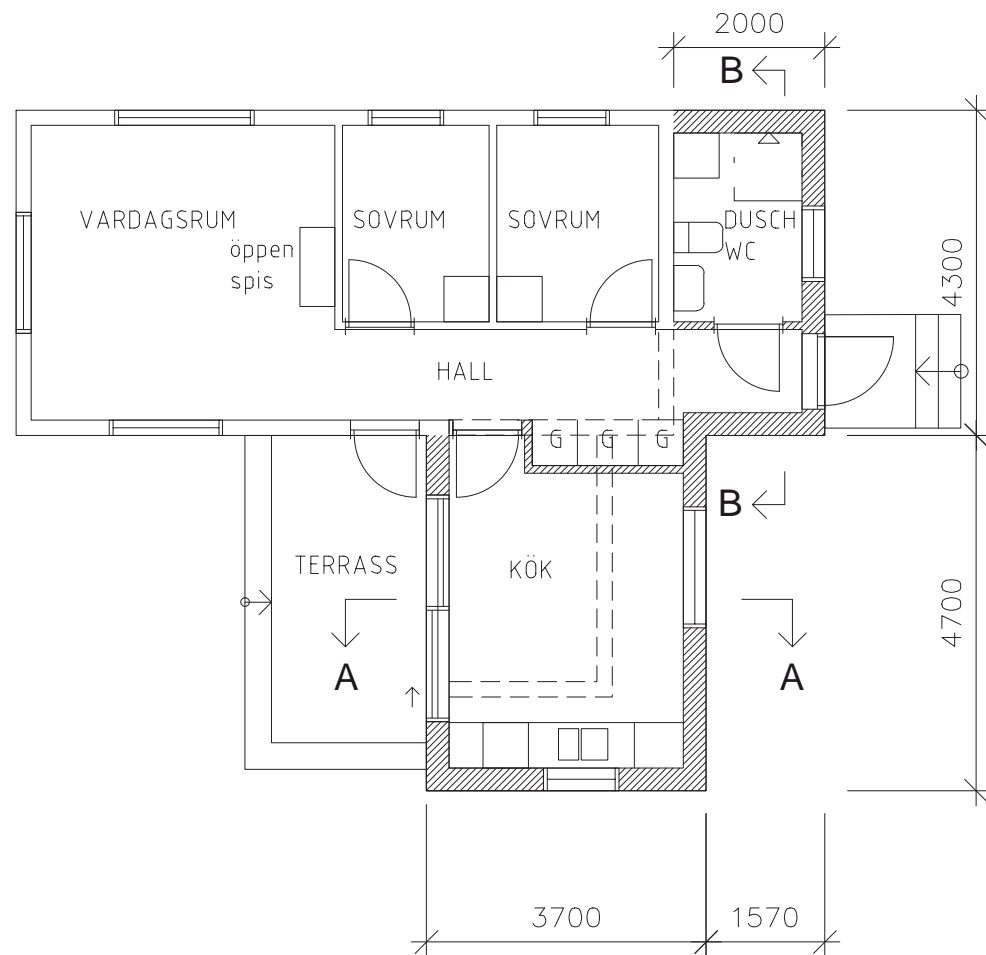
PLAN SKALA 1:100
